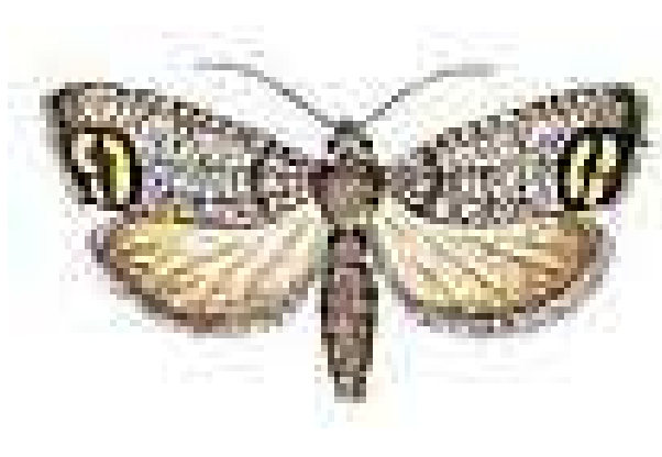
Abbildung 2 Gezeichnete Darstellung eines Apfelwicklers
